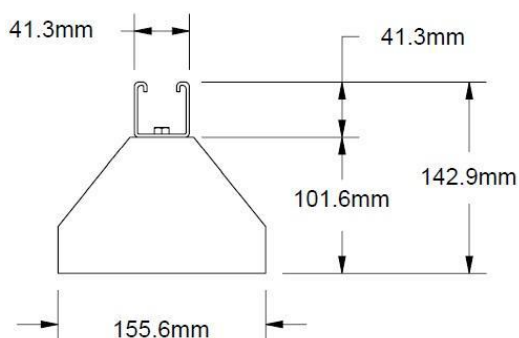
CLI04428 : SUPPORT DE CLIM FOOTBLOC 600 (Charge maxi 300kg)
