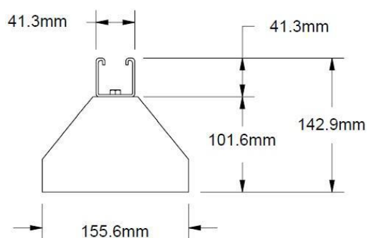
CLI04427 : SUPPORT DE CLIM FOOTBLOC 400 (Charge maxi 300kg)
